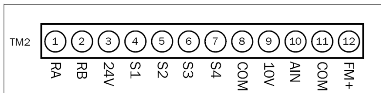
Obr.4 Řídicí svorkovnice
